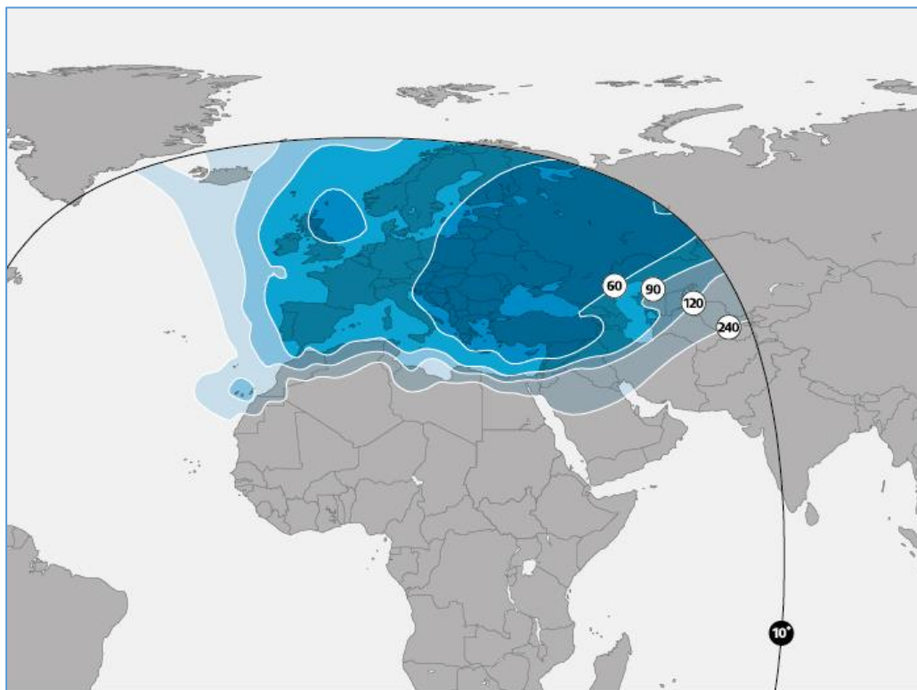
Мапа покриття супутника «Astra 4A»
