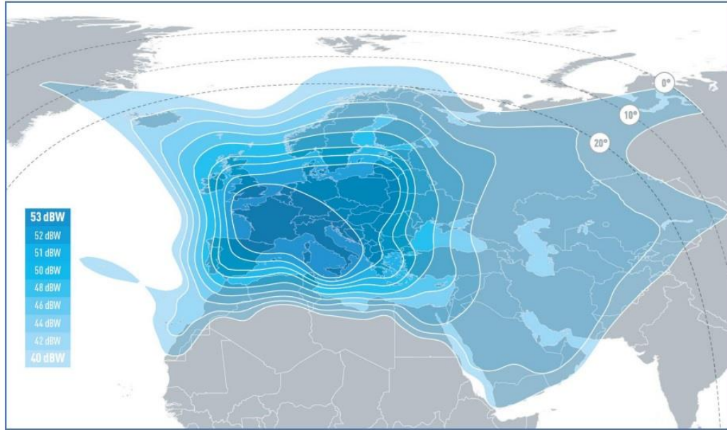
HOTBIRD™ 13G Ku Band Widebeam Downlink Coverage in dBW Мапа покриття супутника «Hot Bird 13G»
